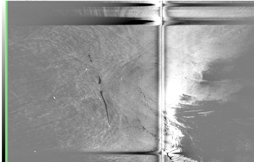
Imagen SLAR que vincula la mancha al buque VEMAOIL XXI
